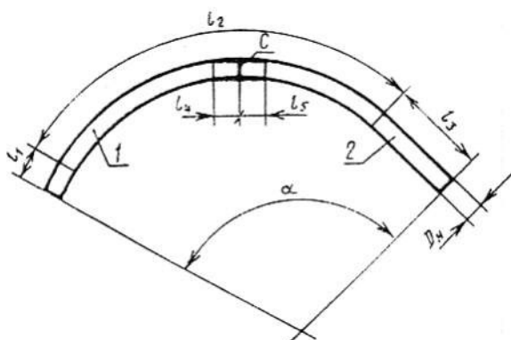
Отвод типа 3
